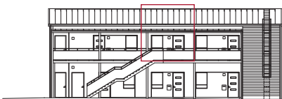
ENTRÉFASAD - ÖST
