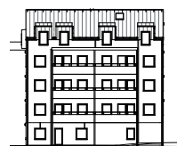
FASAD MOT SYDÖST
