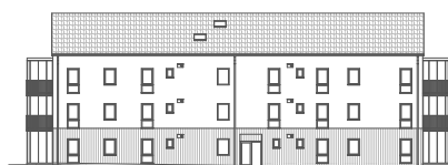
FASAD MOT VÄSTER
